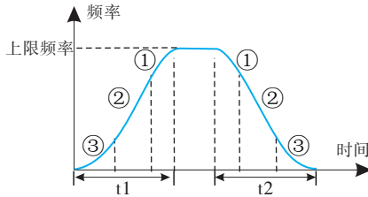
6-04 S曲线加减速
