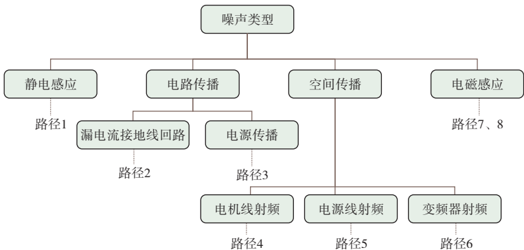
图3-13 噪声分类表
