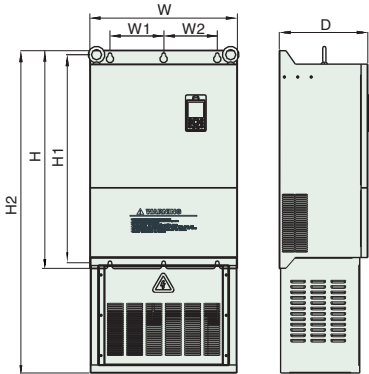
图2-8 加底座
