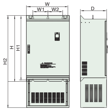
图2-10 加底座
