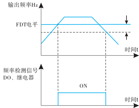
图6-08 FDT功能的电平示意图
