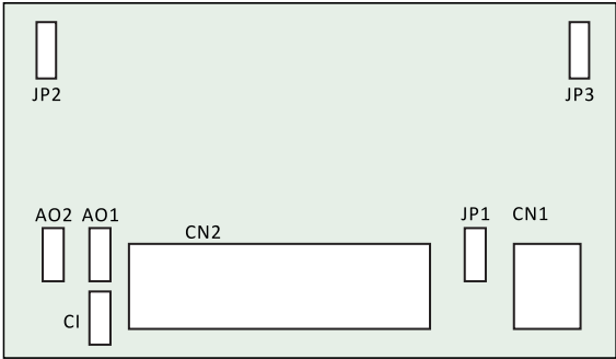
图3-5 控制板端子跳线位置示意图
