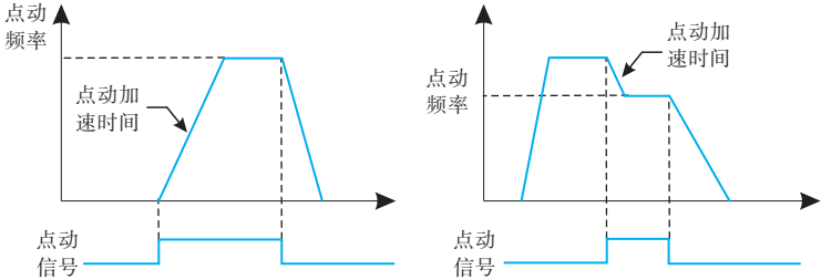
图6-05 点动运行
