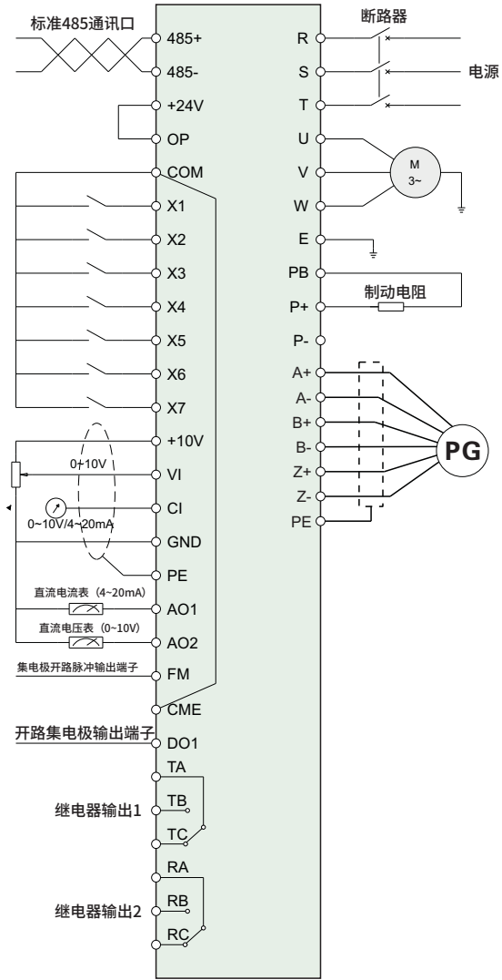
图3-6 基本配线图 (V9-4T0300G,V9-4T0370G)
